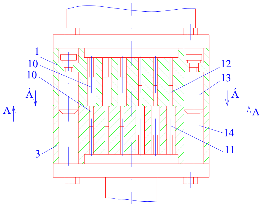
Рисунок 1 – Фронтальний розріз стикувального пристрою
