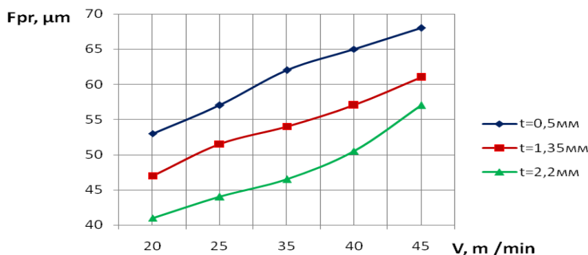
Рисунок 4 – Залежність накопиченої похибки колового кроку від швидкості для S=2,5 мм/об
