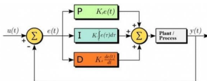
Рисунок 2 – Блок схема ПІД регулятора
