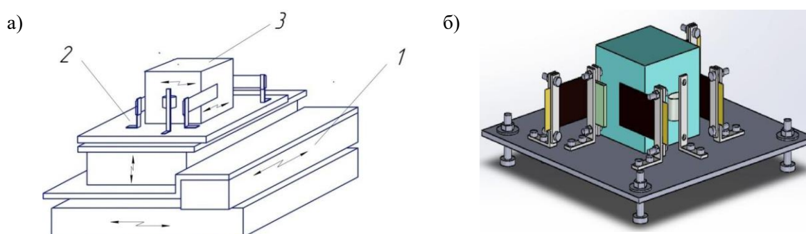
Рисунок 11 – Багатокоординатна система операційного столика комплексу для дослідження мікрооб'єктів (а) і 3D-модель модуля точних переміщень (б): 1 – модуль грубих переміщень, 2 – модуль точних переміщень, 3 – столик
