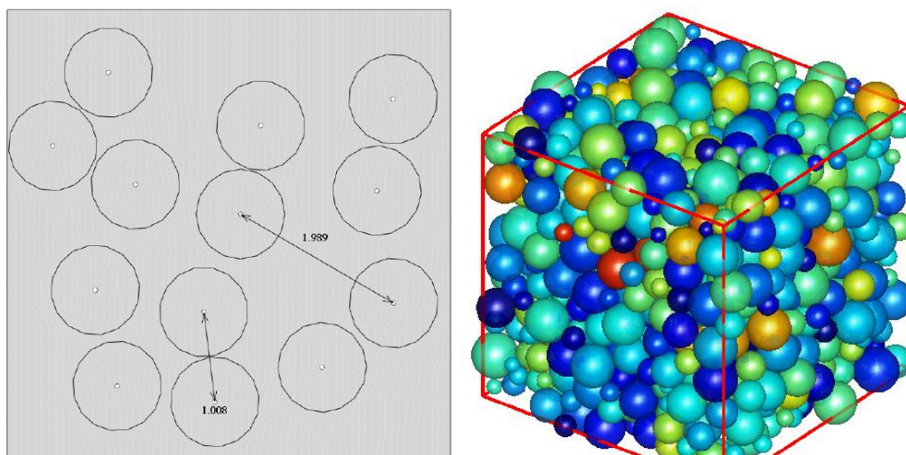
Рисунок 2 – Модель випадкової пористості, яка згенерована в Abaqus з використанням Python
