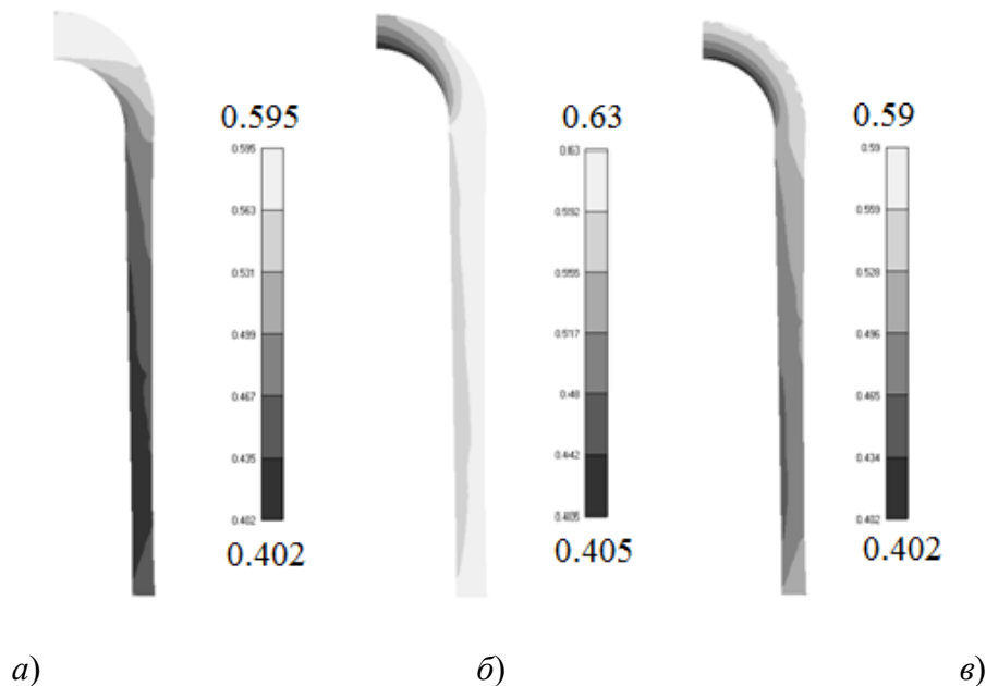
Рисунок 4 – Розподіл пористості при радіальному (а), осьовому (б), радіальному та осьовому (в) ущільненні
