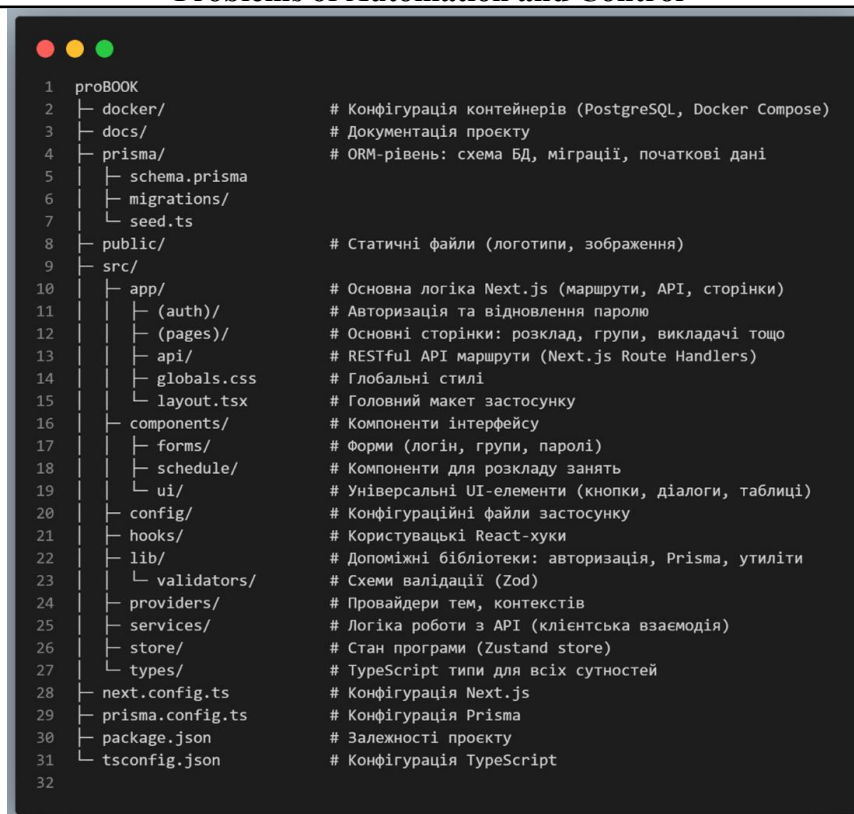
Рис. 1. Основна файлова структура проекту ProBook
