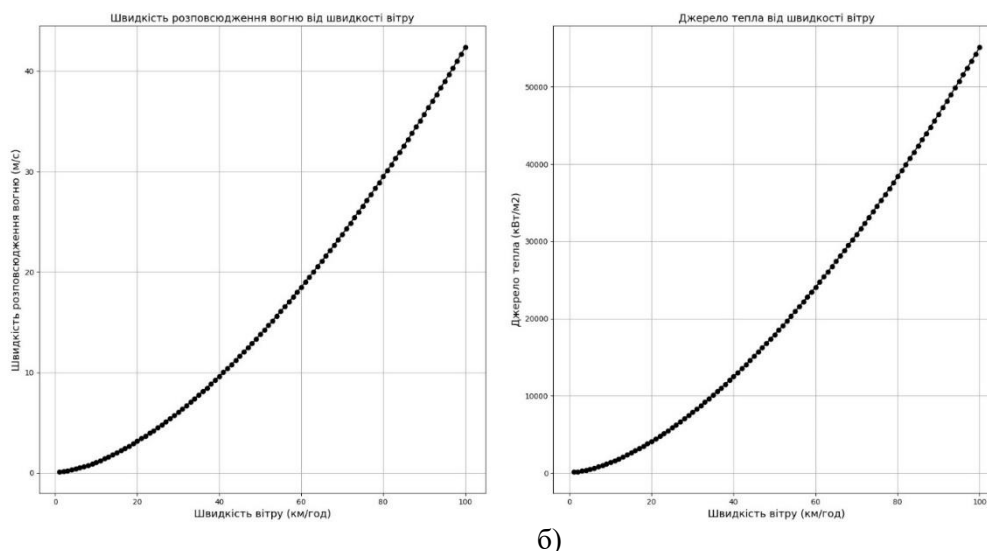
Рисунок 1 – Залежності швидкості розповсюдження вогню та джерела тепла від швидкості вітру
