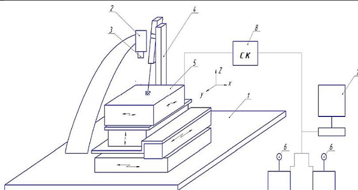
Рисунок 10 – Схема автоматизованого комплексу для дослідження мікрооб'єктів
