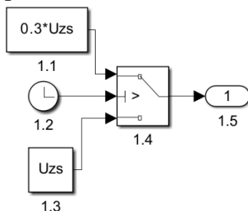
Рисунок 2 – Структурна схема блоку завдання швидкості (1)
