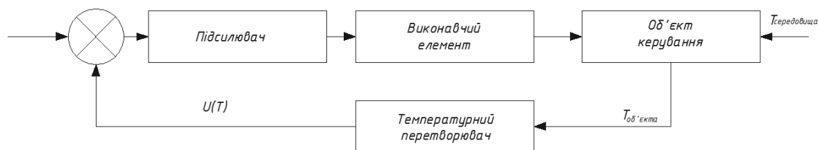
Рисунок 1 – Узагальнена схема термостатування зі зворотним зв'язком
