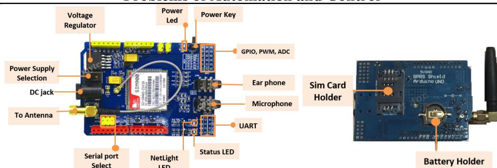
Рисунок 1 – Модуль GSM/GPRS Shield на базі SIM900/800 [6]
