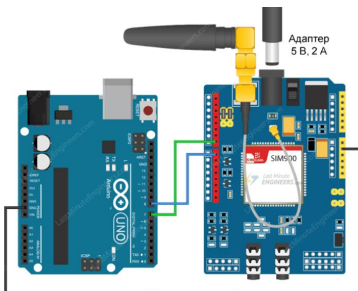
Рисунок 2 – Схема підключення модуля до плати Arduino [7]
