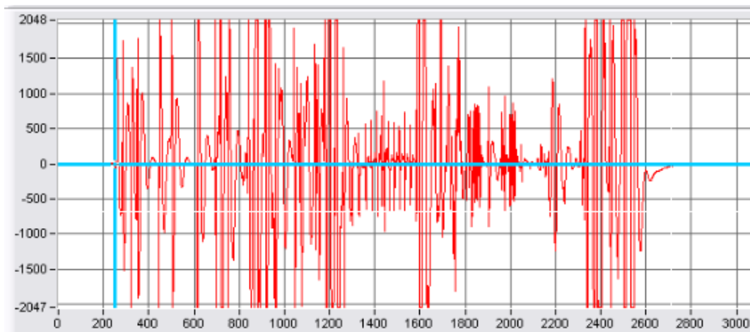
Рисунок 3 – Форма сигналу акустичної емісії
