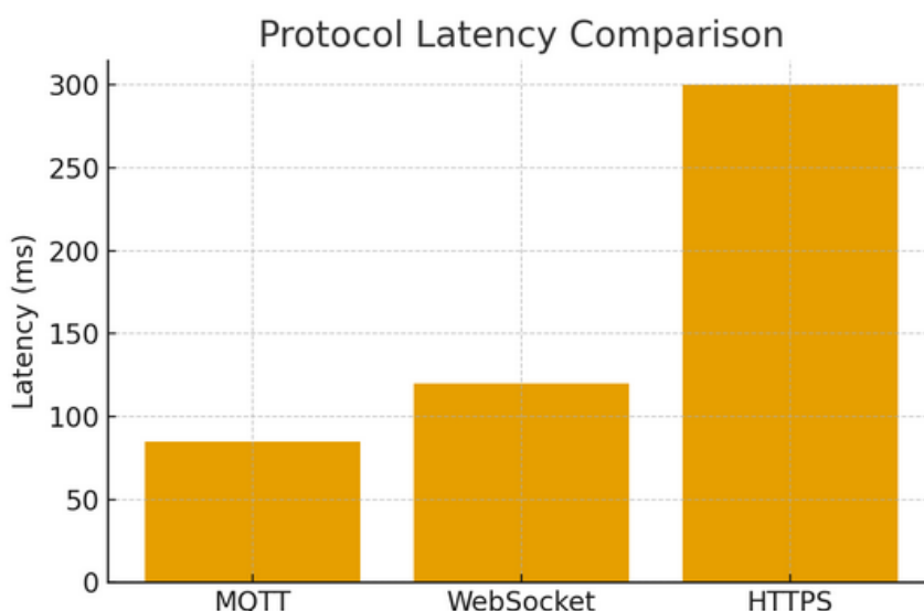
Рисунок 2 – Порівняльна діаграма затримок протоколів MQTT, HTTPS та WebSocket
