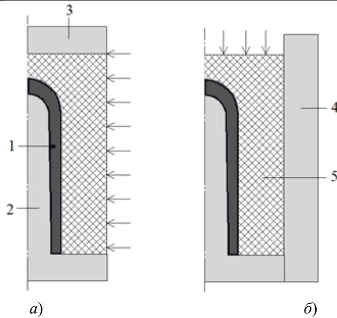
Рисунок 3 – Схеми радіального (а) та осьового (б) ущільнення фільтруючого елемента складної форми у вигляді колби: 1 - порошок, що ущільнюється; 2 - оправка; 3 - кришка; 4 - стінка; 5 - еластичний елемент
