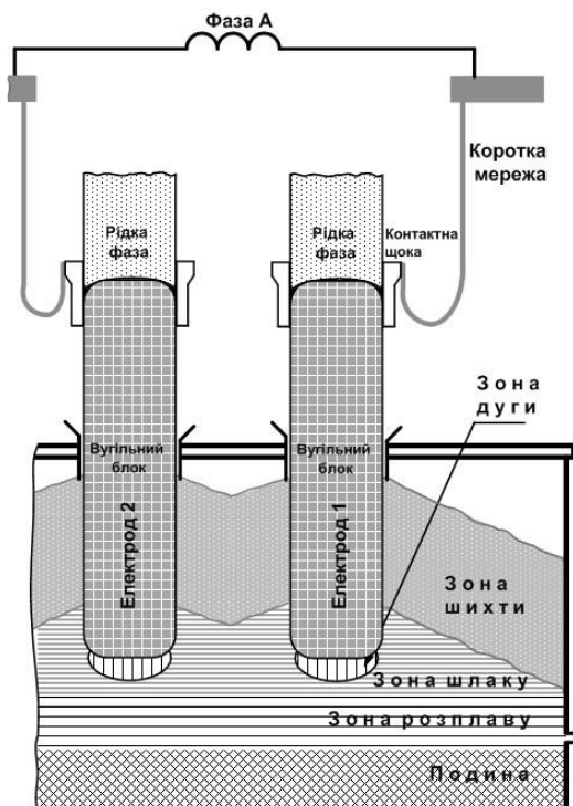
Рис.2. Переріз ванни печі РПЗ-63 (одна фаза)
