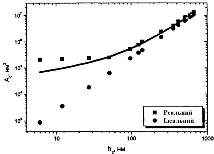
Рисунок 3 – Співвідношення між глибиною та площею проекції контакту для ідеального та реального інденторів. Матеріал – плавлений кварц
