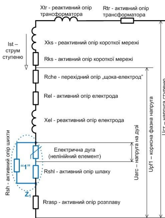
Рис.3. Схема заміщення (один електрод)
