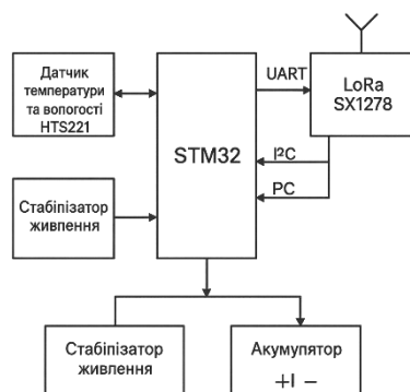
Рисунок 1 – Структурна схема розробленого комунікаційного пристрою
