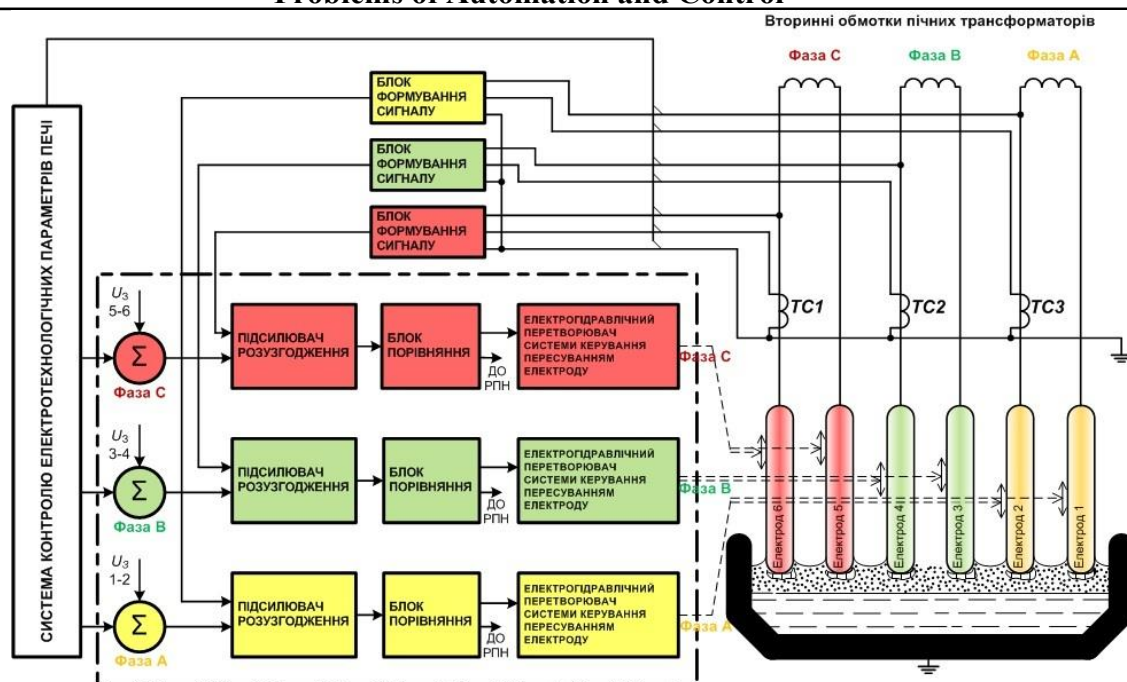
Рис. 4. Спрощена структурна схема системи керування піччю РПЗ-63
