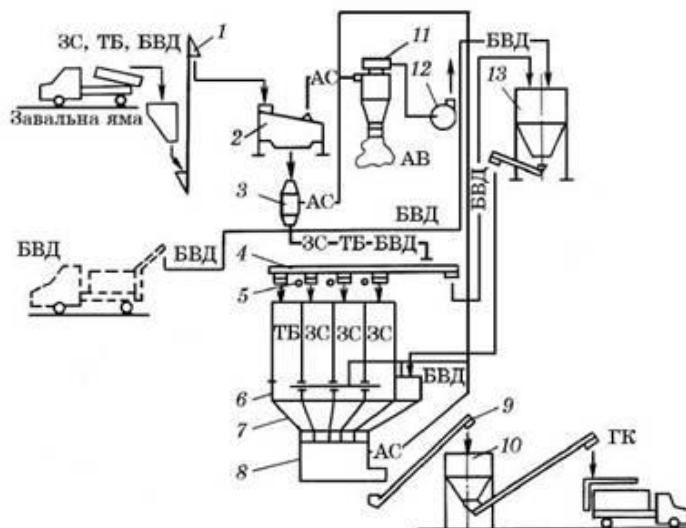
Рисунок 1 – Технологічна схема виробництва комбікормів агрегатом УМК-Ф-2:
