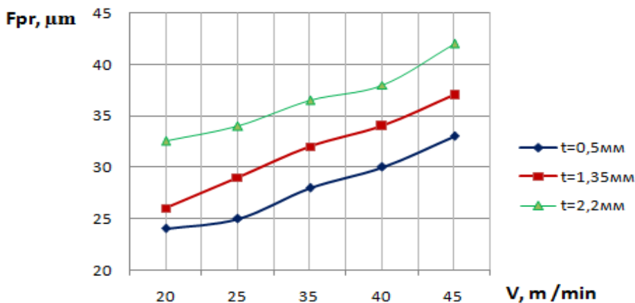
Рисунок 3 – Залежність накопиченої похибки колового кроку від швидкості для S=0,5 мм/об
