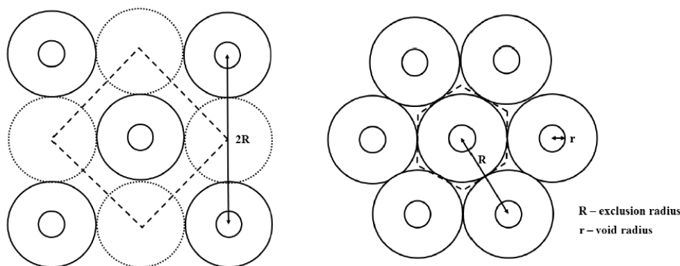
Рисунок 1 – Варіанти конфігурації упаковок створених в Abaqus
