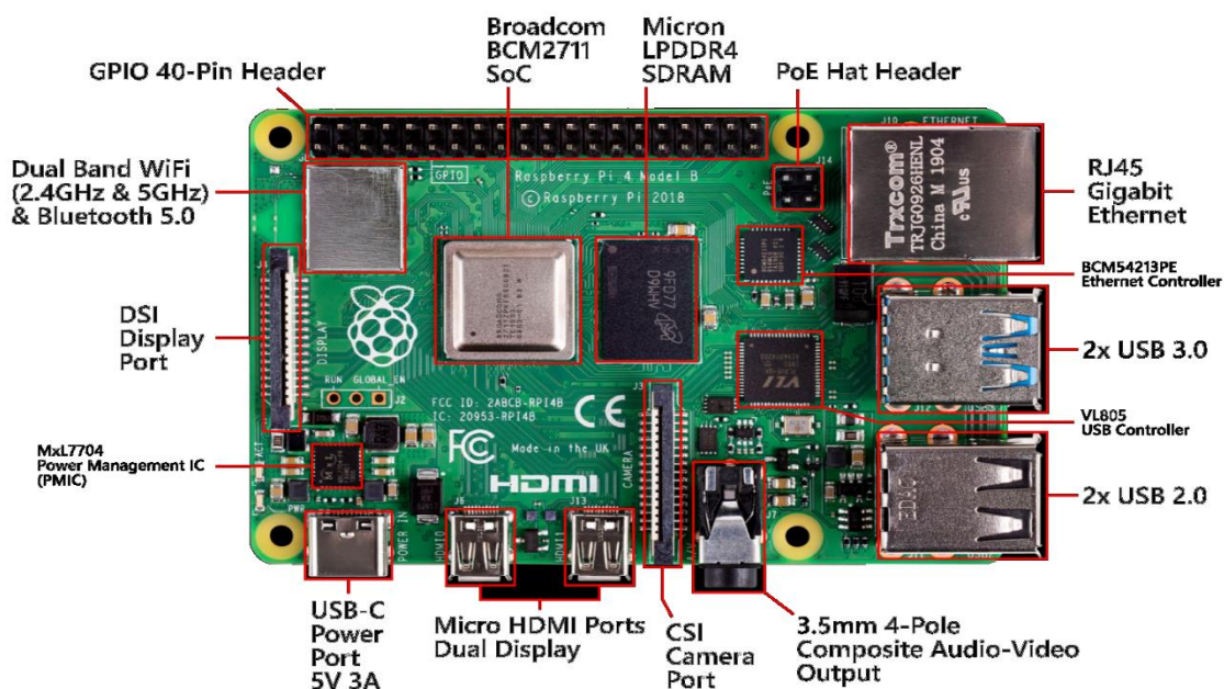
Рисунок 1 – Типовий вигляд плати Raspberry Pi 4
