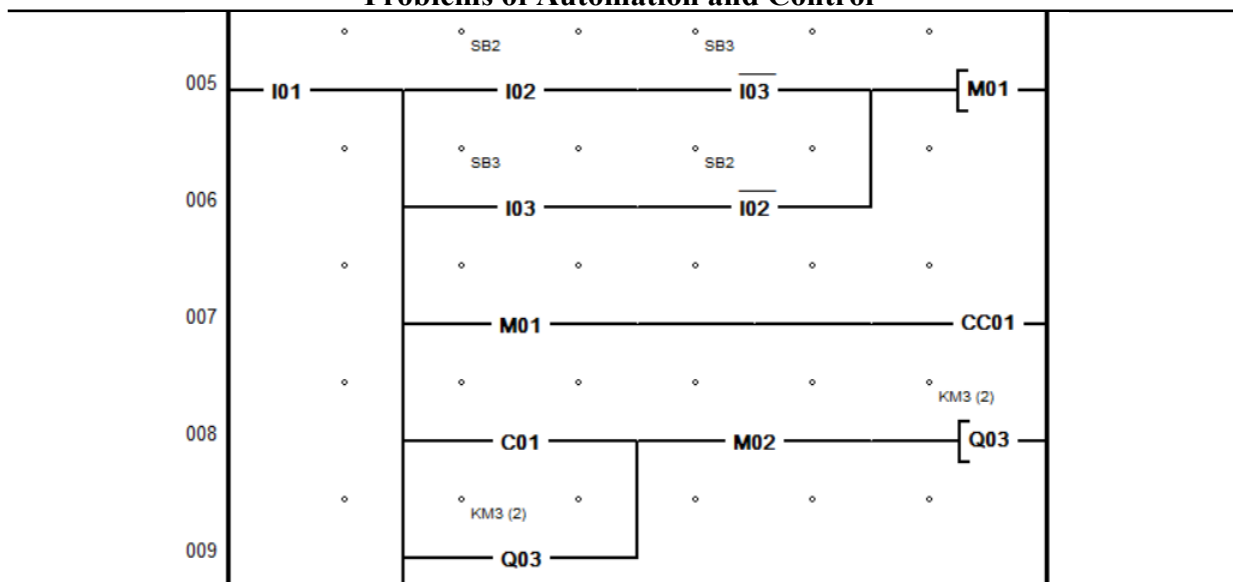
Рисунок 5 – Програма керування асинхронним двигуном з фазним ротором від програмованого реле EASY 512-DC-RC (пуск на другій пусковій ступені)
