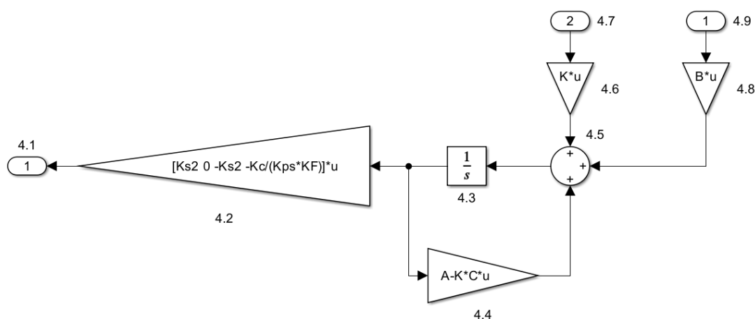
Рисунок 4 – Підсистема System (4) спостерігача
