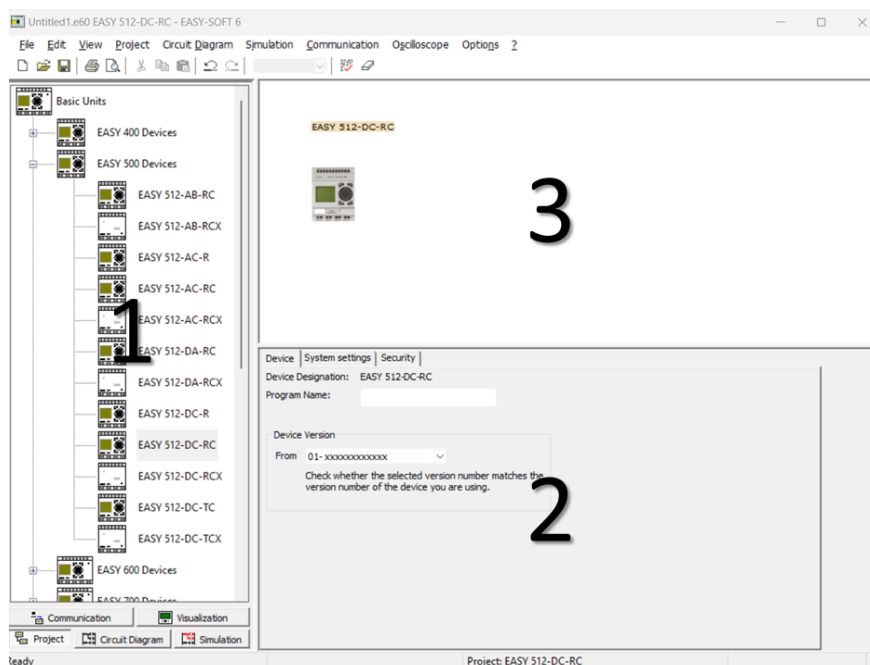
Рисунок 4 – Інтерфейс EASY-SOFT 6 в режимі «Проект»
