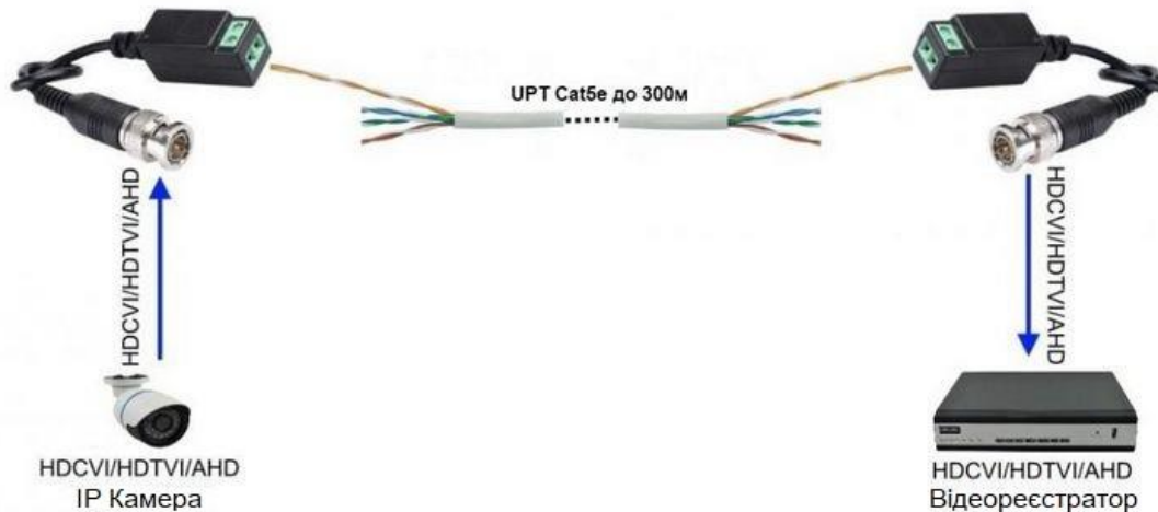
Рисунок 3 – Підключення системи відеоспостереження по витій парі
