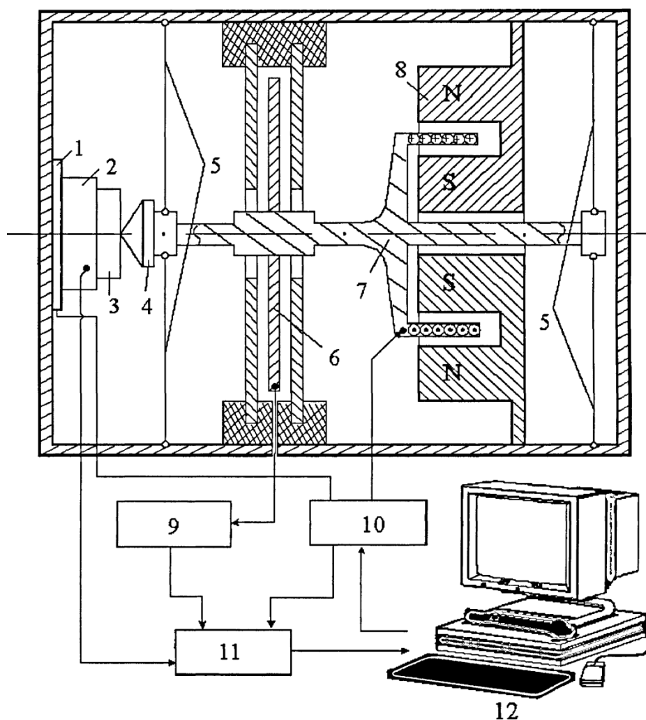
Рисунок 1 – Блок-схема експериментальної установки для динамічного наноіндентерування. 1 – столик з 3-х координатним п'єзокерамічним приводом, 2 – датчик навантаження, 3 – зразок, 4 – індентор, 5 – елементи підвісу, 6 – ємнісний датчик зміщення, 7 – котушка електромагнітного приводу, 8 – постійний магніт, 9 – підсилювач і підсилювач потужності, 11 – аналого-цифровий перетворювач, 12 – комп'ютер, 13 – станина
