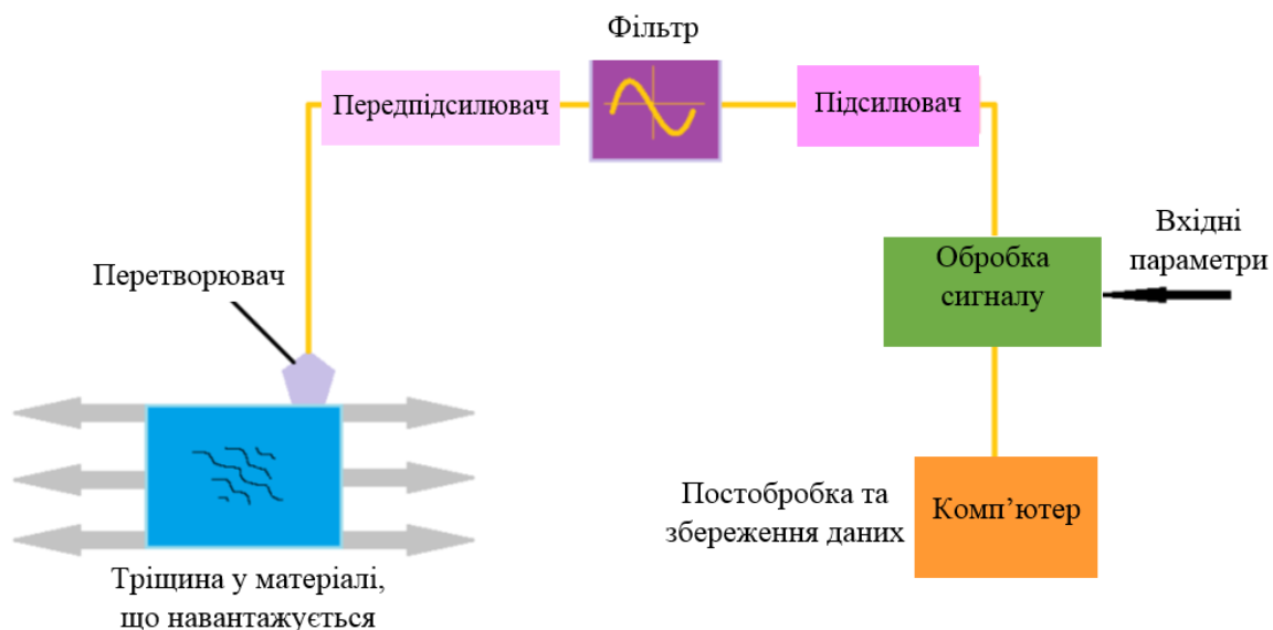
Рисунок 1 – Схема вимірювання параметрів акустичної емісії
