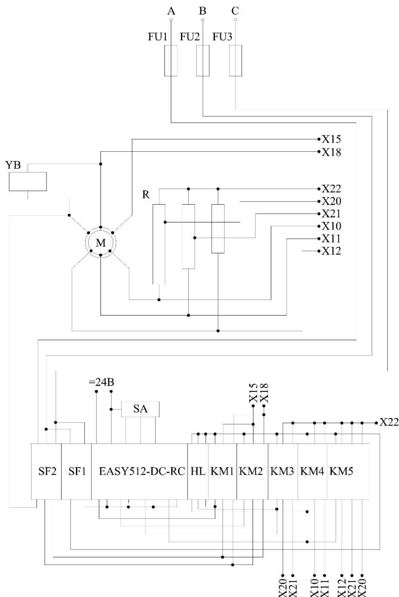
Рисунок 3 – Схема електрична принципова проектна
