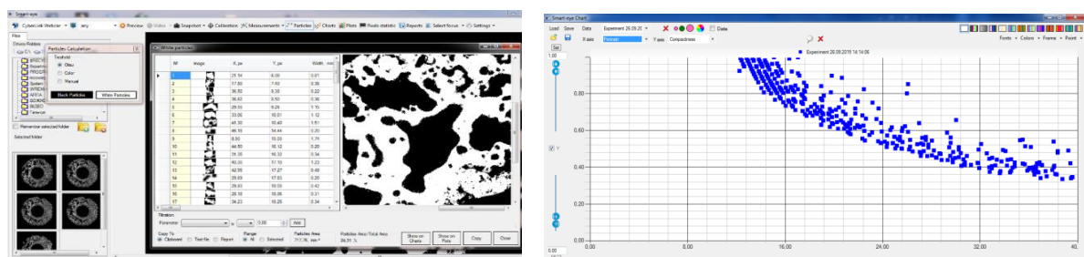
Рисунок 3 – Аналіз розподілу пористості ППМ здійснювався за допомогою прикладної програми Smart-eye
