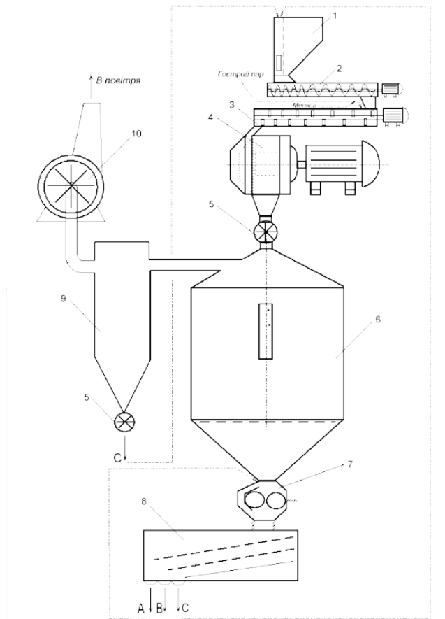
Рисунок 2 – Принципова схема лінії гранулювання:
