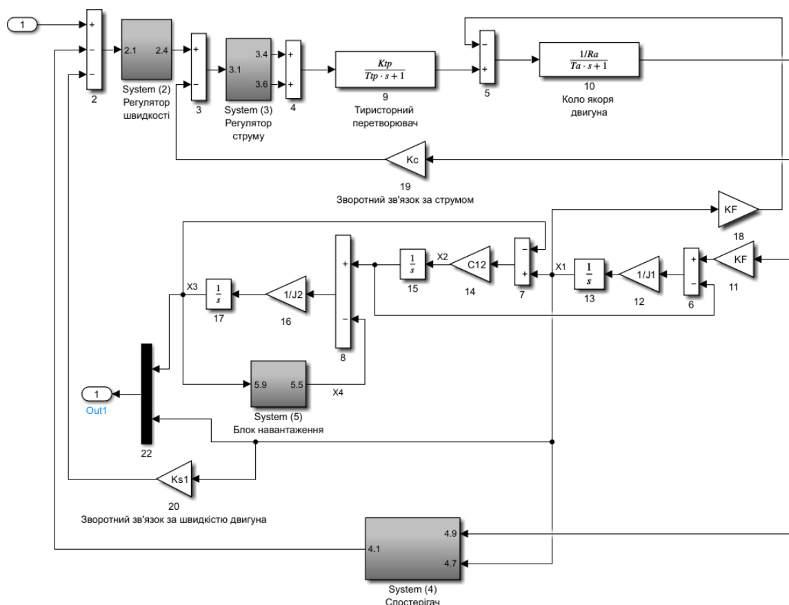
Рисунок 3 – Структурна схема моделі електропривода (2)
