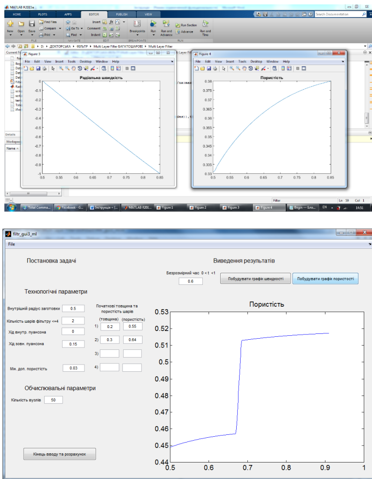
Рисунок 3 – Виведення графічних залежностей впливу радіальної швидкості та розподілу пористості при моделюванні радіально-ізостатичного пресування багатoshарового ППМ
