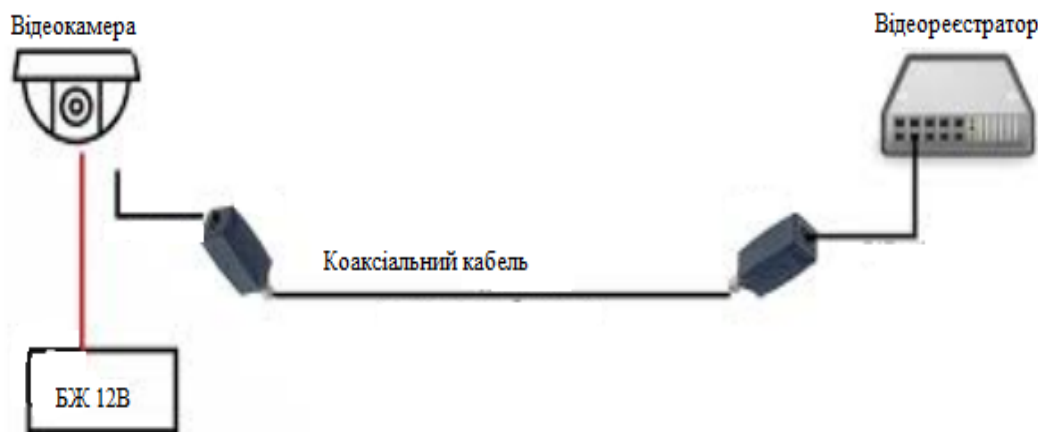
Рисунок 2 – Схематичне зображення підключення аналогової системи
