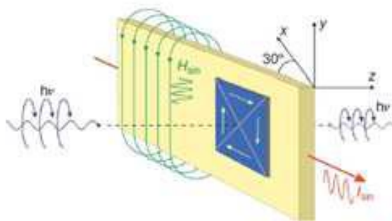
Рисунок 1 – Схема дослідів вивчення перемикання полярності вихрового ядра [1]
