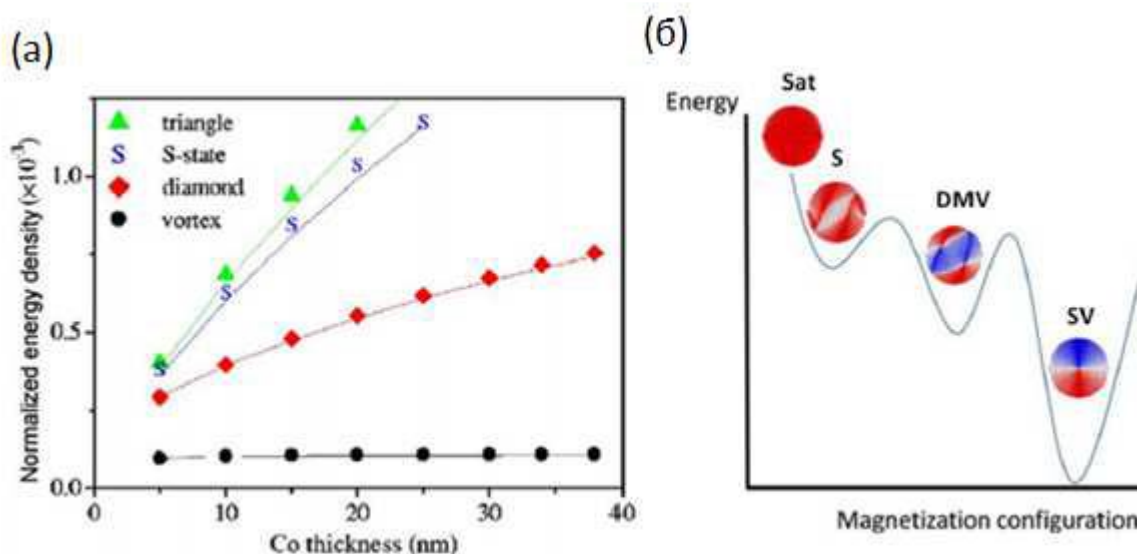
Рисунок 3 – (а) залежність щільності магнітної енергії від товщини для Co циліндрів діаметром 1,65 мкм. (б) схематичне зображення енергії в різних МС та основного стану (SV) [1]
