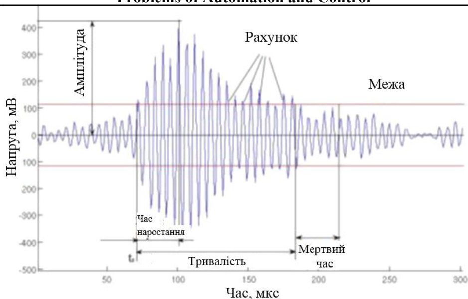
Рисунок 2 – Визначення параметрів дискретного сигналу
