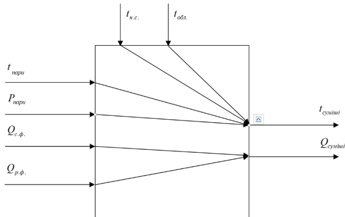
Рисунок 3 – Структурна схема взаємозв'язків технологічних параметрів об'єкта: Q_{с.ф.} – витрата сухих компонентів; Q_{р.ф.} – витрата рідких компонентів; t_{парі} – температура перегрітої пари; P_{парі} – тиск пари; t_{суміші} – об'єм гранул; Q_{суміші} – температура гранул; t_{н.с.} – температура навколишнього середовища; t_{обл.} – температура частин обладнання.
