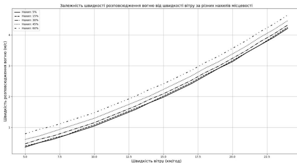
Рисунок 2 – Залежність швидкості розповсюдження вогню від швидкості вітру за різних нахилів місцевості
