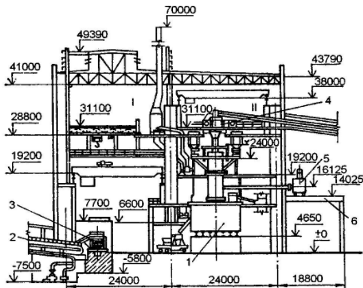
Рис.1. Розріз цеху виробництва марганцевих феросплавів НЗФ з печами РПЗ-63:
