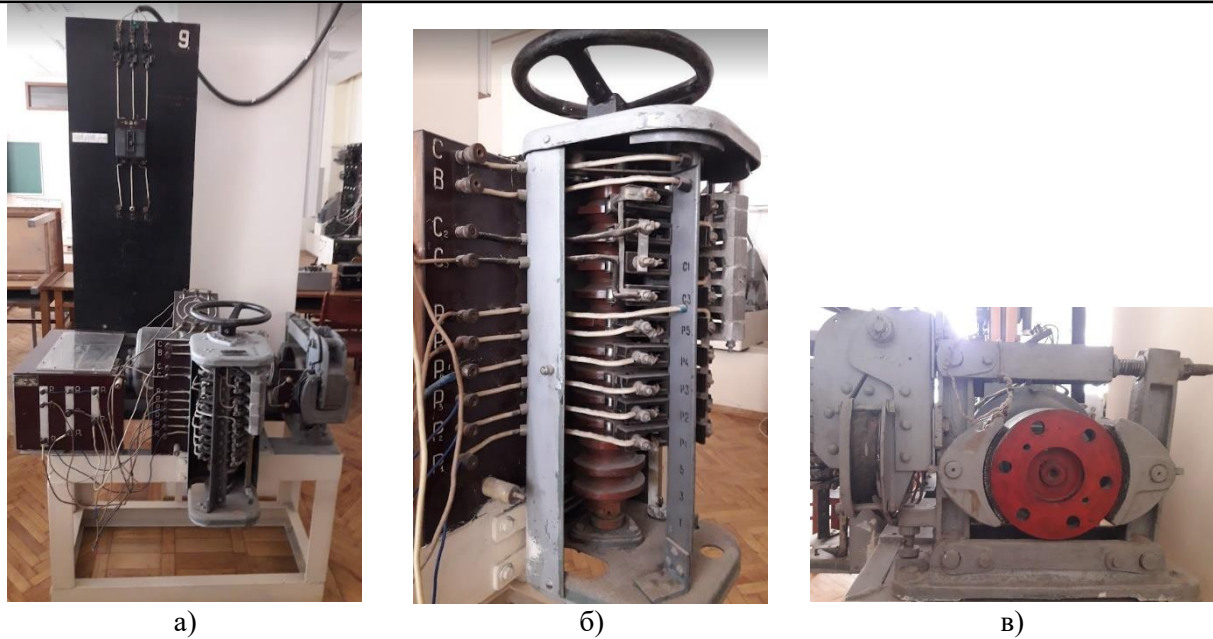
Рисунок 1 – Загальний вигляд стенду в базовому варіанті (а), контролеру НТ-51 (б) та колодкового гальма двигуна (3)
