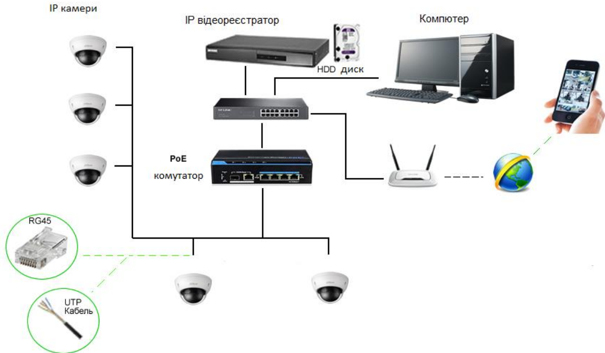
Рисунок 5 – Схема Ір-відеоспостереження
