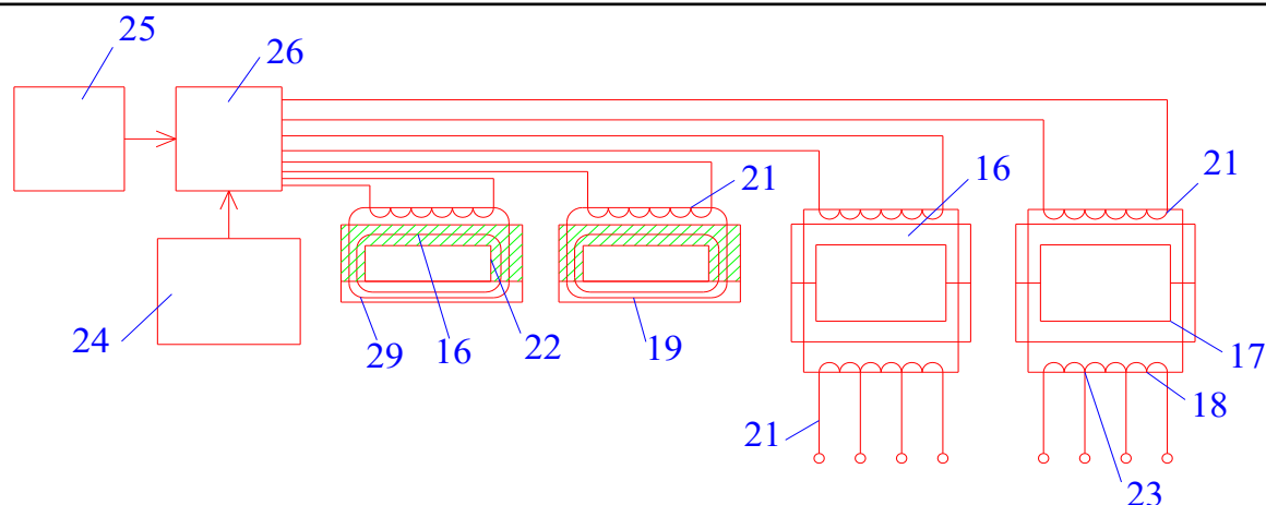
Рисунок 5 – Схема пристрою з роздільною передачею електричної енергії
