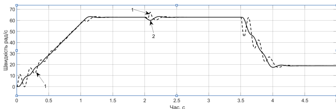
Рисунок 5 – Графіки перехідних процесів за кутовою швидкістю двигуна (1) та механізму (2) для математичної моделі зі спостерігачем
