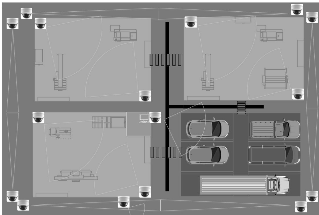
Рисунок 7 – Схема розташування камер на підприємстві.
