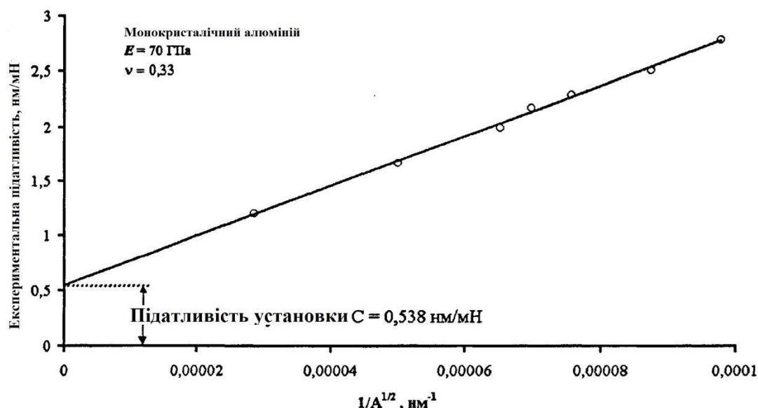
Рисунок 2 – Залежність підатливості C_{\text{total}} системи «зразок – установка» від розміру відбитку для монокристалічного А1
