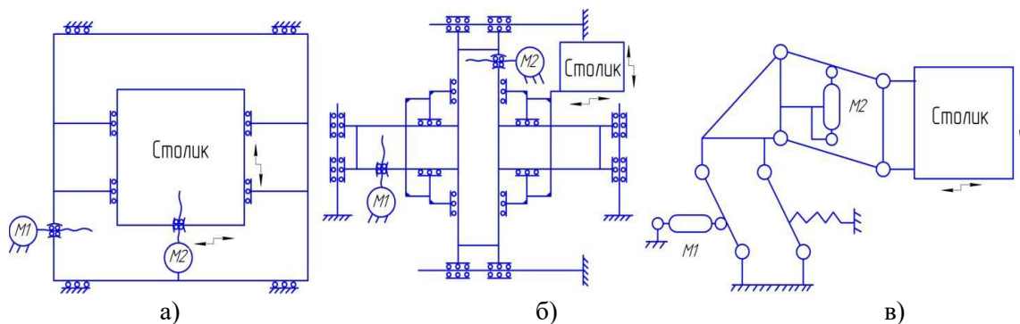
Рисунок 9 – Кінематичні схеми двокоординатних систем плоскопаралельного руху для точного позиціонування: а – послідовна з поступальними напрямними; б – паралельна з прогресивними напрямними; в – послідовна з шарнірами
