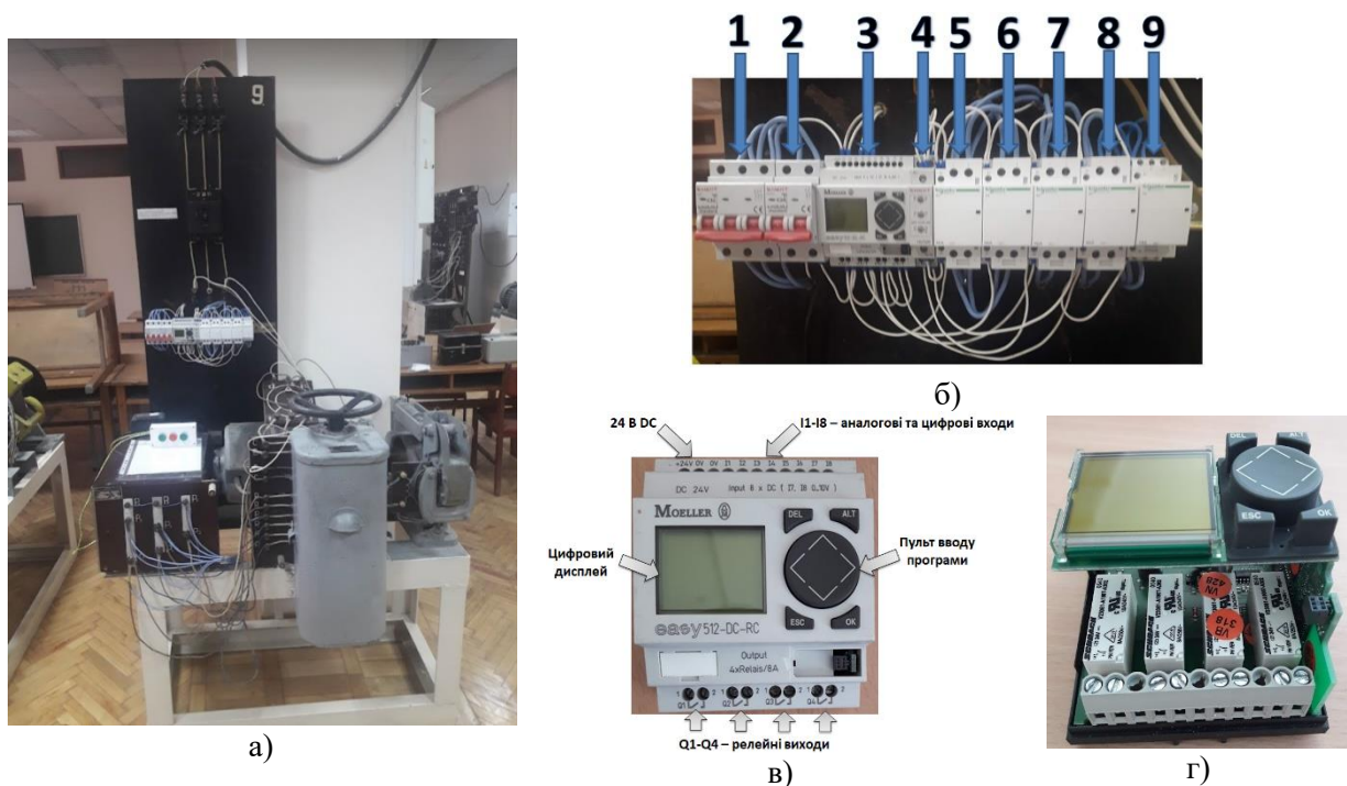
Рисунок 2 – Загальний вигляд стенду в проектному варіанті (а), апаратури керування двигуном (б) та електронного реле з його складовими елементами (в, г)
