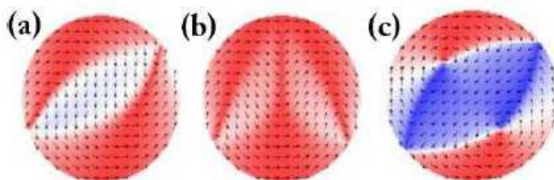
Рисунок 2 – Метастабільні стани: (а) S-стан; (b) Т-стан (с) Подвійний вихровий стан [2]
