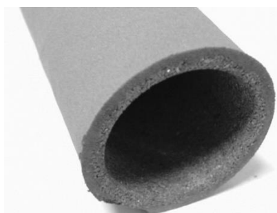
Рисунок 1 – Багат шаровий ППМ з порошку сталі ШХ15 Ø40×220 мм виготовлений методом радіально-ізостатичного пресування
