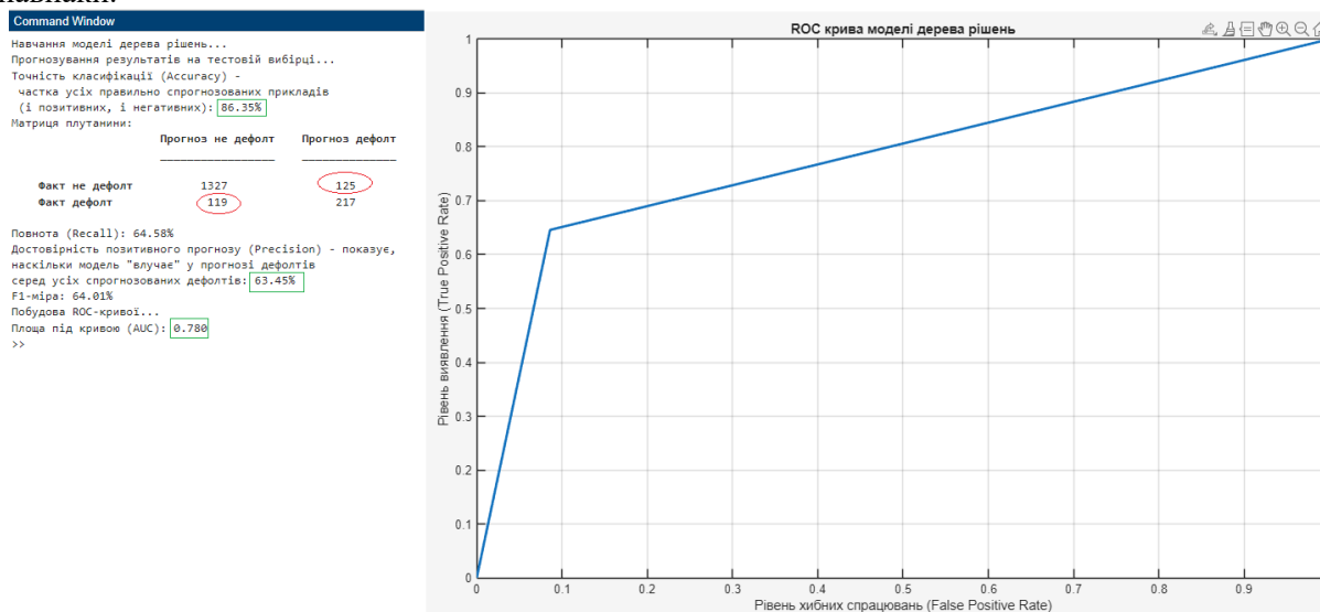
Рис. 1. Результат моделі з передбачення дефолту на датасеті HMEQ, побудованої в MATLAB
