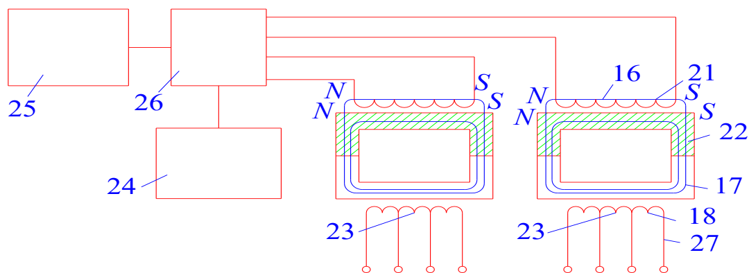
Рисунок 4 – Схема пристрою при роботі в режимі максимального зусилля
