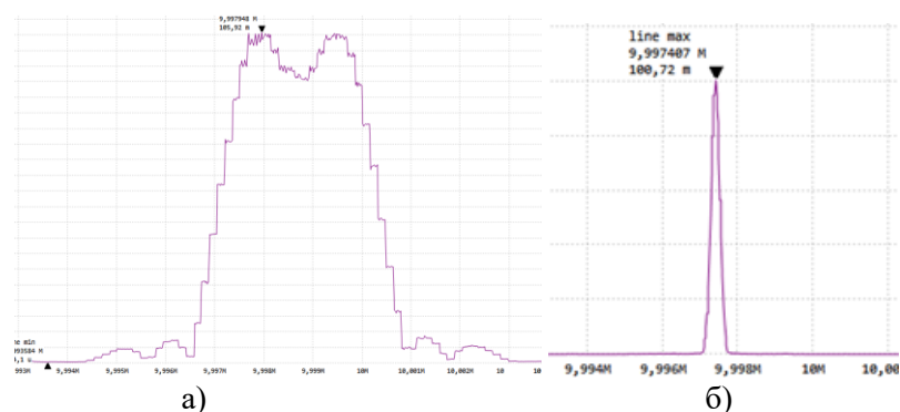
Рис. 1. Порівняння спектрального відгуку резонатора: а) TinySA, RBW=3000 Гц; б) TinySA Ultra, RBW=200 Гц
