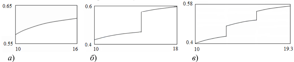
Рисунок 2 – Розподіл пористості по радіусу (мм) в одношаровому (а), двошаровому (б) і тришаровому (в) фільтруючих елементах
